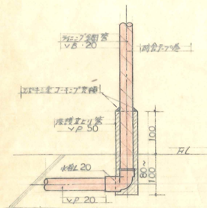
給水管立上り S=1:5
